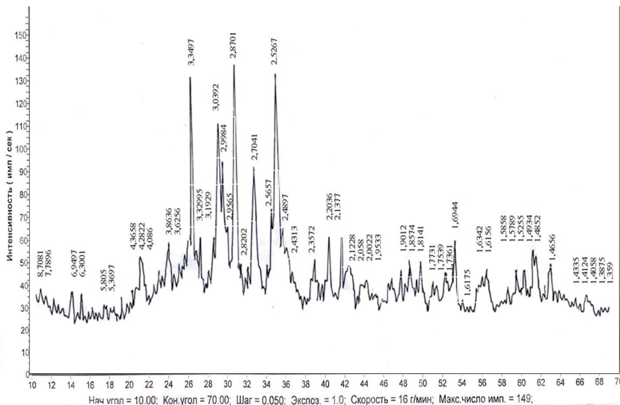
Сурет 3 - Ащысай металлургия зауытында мырышты кендерді вельцилеу процесінен алынған клинкердің рентгенограммасы
