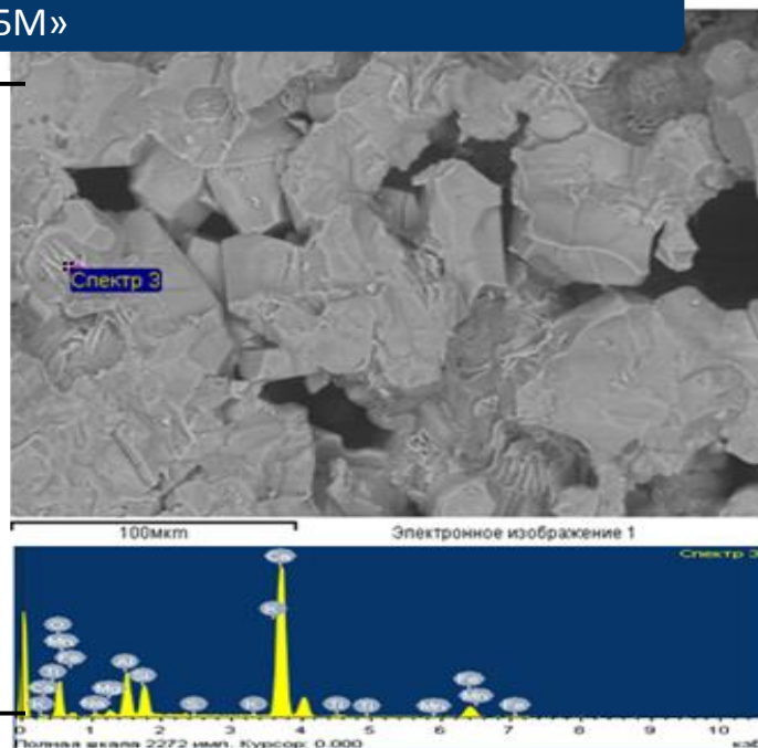
Сурет 12 - 1350 °C температурада күйдірілген № 4 клинкердің құрылымы және құрамы C 4 AF, электронды-микроскопиялық талдау деректері бойынша
