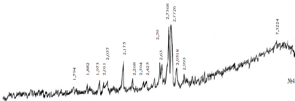
Сурет 11 – 1350 °С температурада күйдірілген «эктас қалдығы + электротермофосфорлы шлак + Ащысай клинкері» шикізат шихтасынан алынған № 4 клинкердің рентгенограммасы
