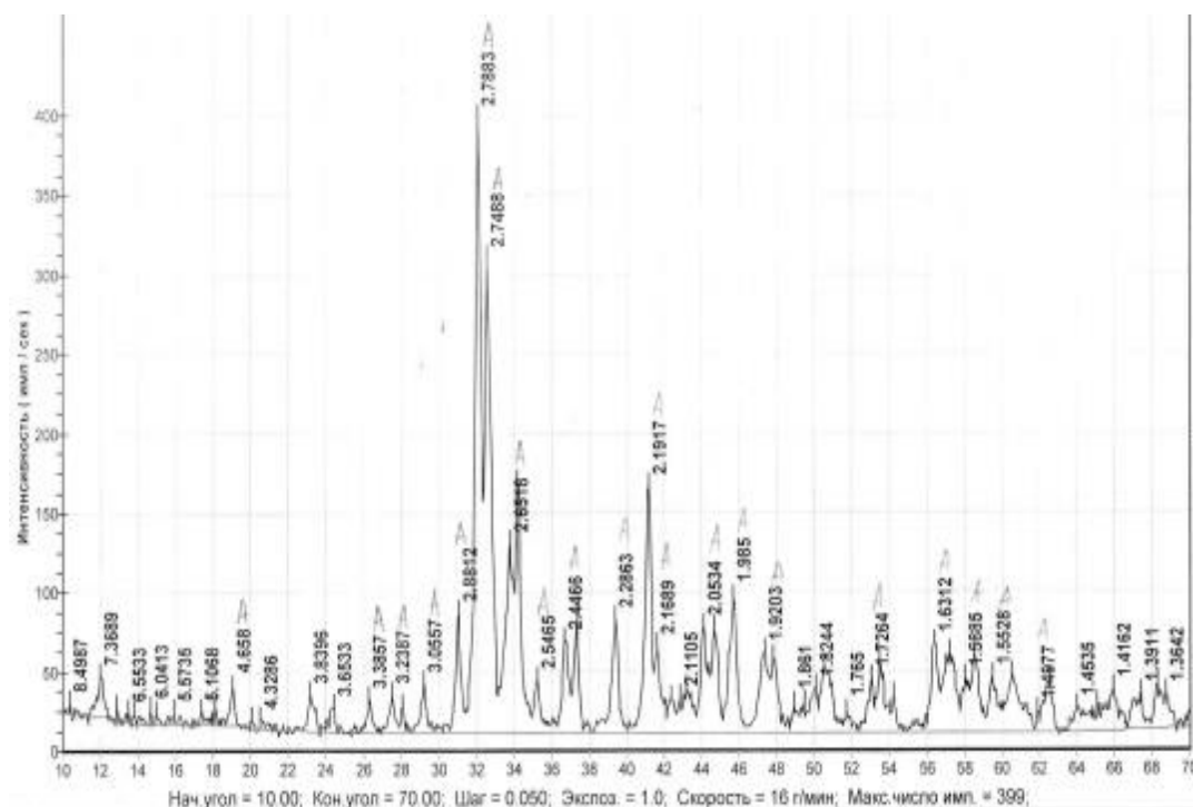
Сурет 15- 1300 °С температурада күйдірілген клинкерлердің ретгенограммалары
